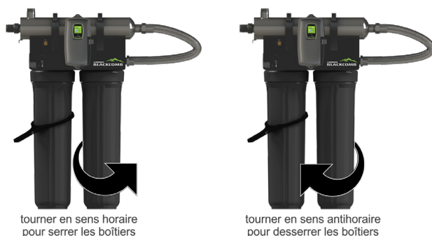
Figure 5. Retrait des cartouches de filtre
